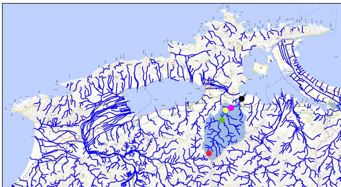
松江・出雲周辺の河川と意宇川流域図（国土数値情報 流域メッシュデータを QGIS により表示）。
